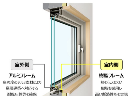
高断熱アルミ樹脂複合窓「EXIMA 55」(構造図解 (左) と施工イメージ (右))
