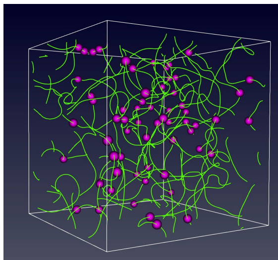
図1:シミュレーションされた量子乱流のスナップショット。緑色の線は量子渦の芯、紫色の球は追従粒子。
