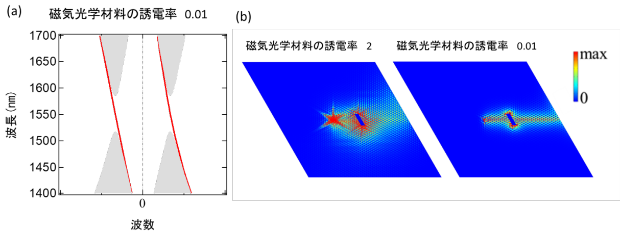
図2(a) カイラルエッジ状態の存在を示す導波路構造の分散関係。赤い曲線がカイラルエッジ状態の分散曲線を示す。(b) 導波路上に欠陥が存在する場合の光伝搬の様子。誘電率が小さいほど、乱れが少なく伝搬している様子がわかる。
