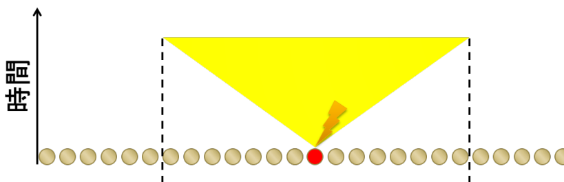
図2 線形光円錐の概要図（1次元）
