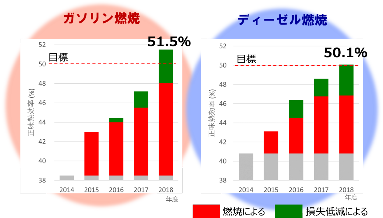
図1 正味最高熱効率50%超達成の推移
