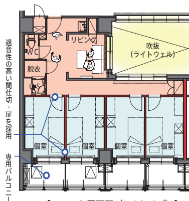
【ユニット平面図 (A-1タイプ)】
