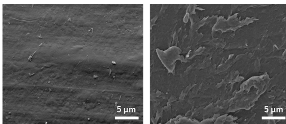
図 1 P-Life 添加 PP ストローの表面の電子顕微鏡画像 未処理のストロー(左)と微生物処理したストロー(右)
