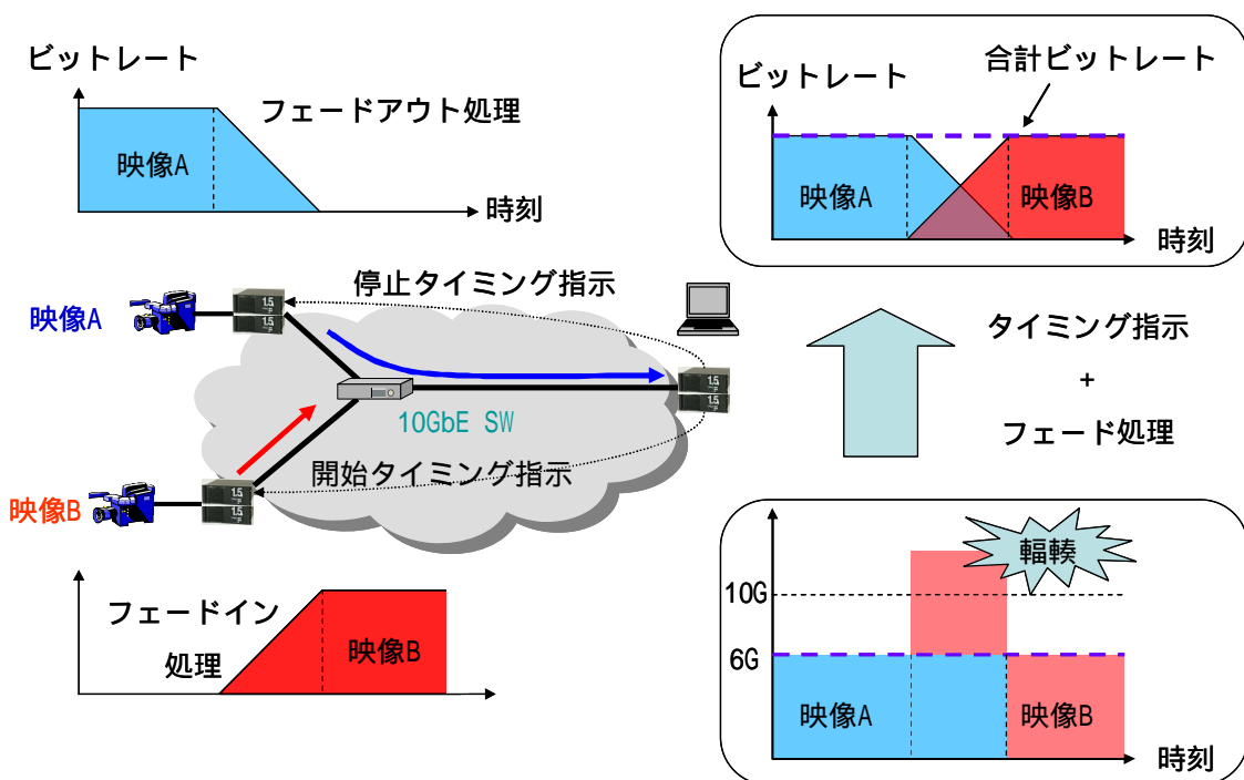
(図3) 非圧縮 4K 映像素材をネットワーク上で切替え編集する技術の概要
